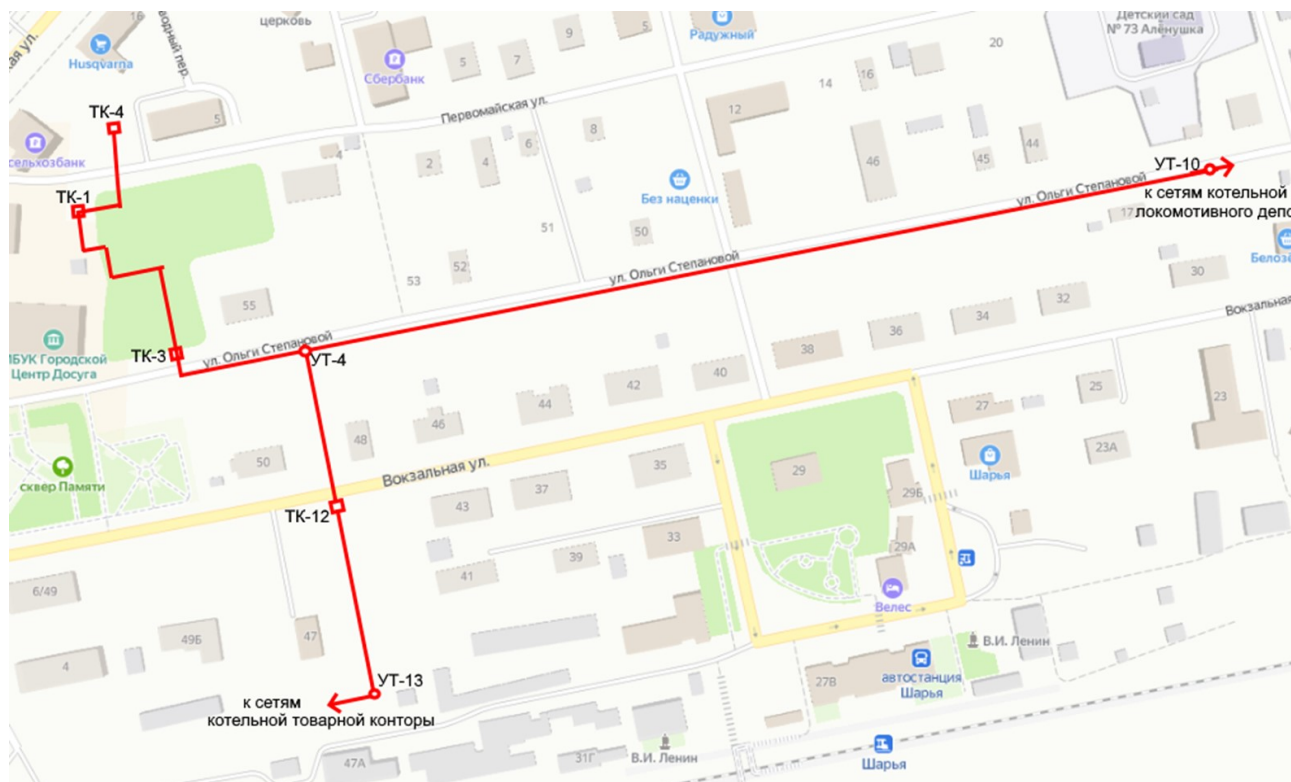
Рисунок 5.3.1 - Схема подключения котельных товарной конторы и локомотивного депо к тепловым сетям Шарьинской ТЭЦ.
