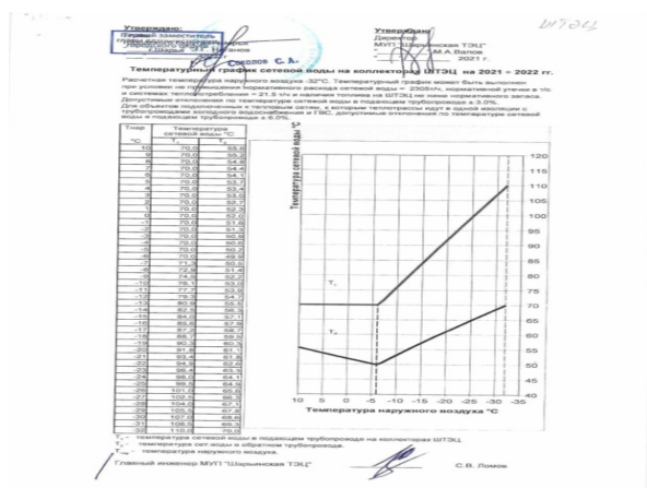
Рисунок 1.3.1 – Температурный график тепловой сети Шарьинской ТЭЦ
