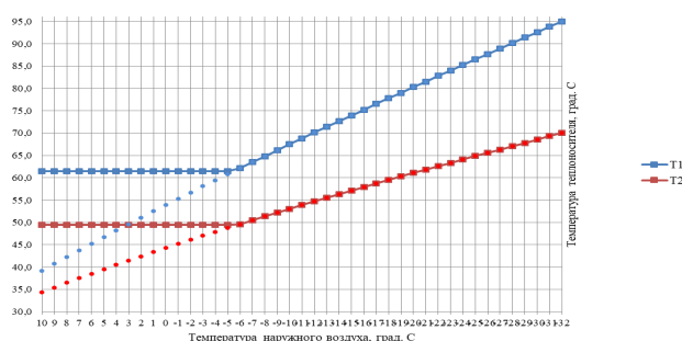
Рисунок 1.3.3 – Температурный график тепловых сетей от котельной локомотивного депо ОАО «РЖД»
