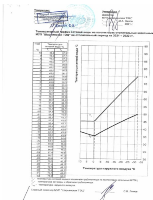
Рисунок 1.3.1 – Температурный график тепловой сети Шарьинской ТЭЦ
