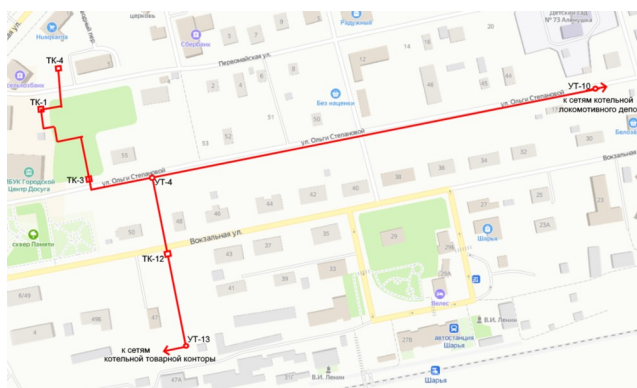
Рисунок 5.4.1 - Схема подключения котельных товарной котормы и локомотивного депо к тепловым сетям Шарьинской ТЭЦ
