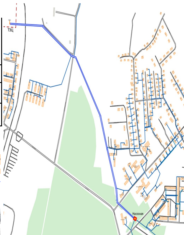
Рисунок 6.5.1 - Схема тепловых сетей от ТЭЦ до города Шарья после прокладки новых тепломагистралей
